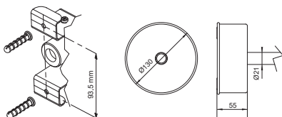
dettagli per le lampade 1800 e 1890 details for 1800 and 1890 lamps
